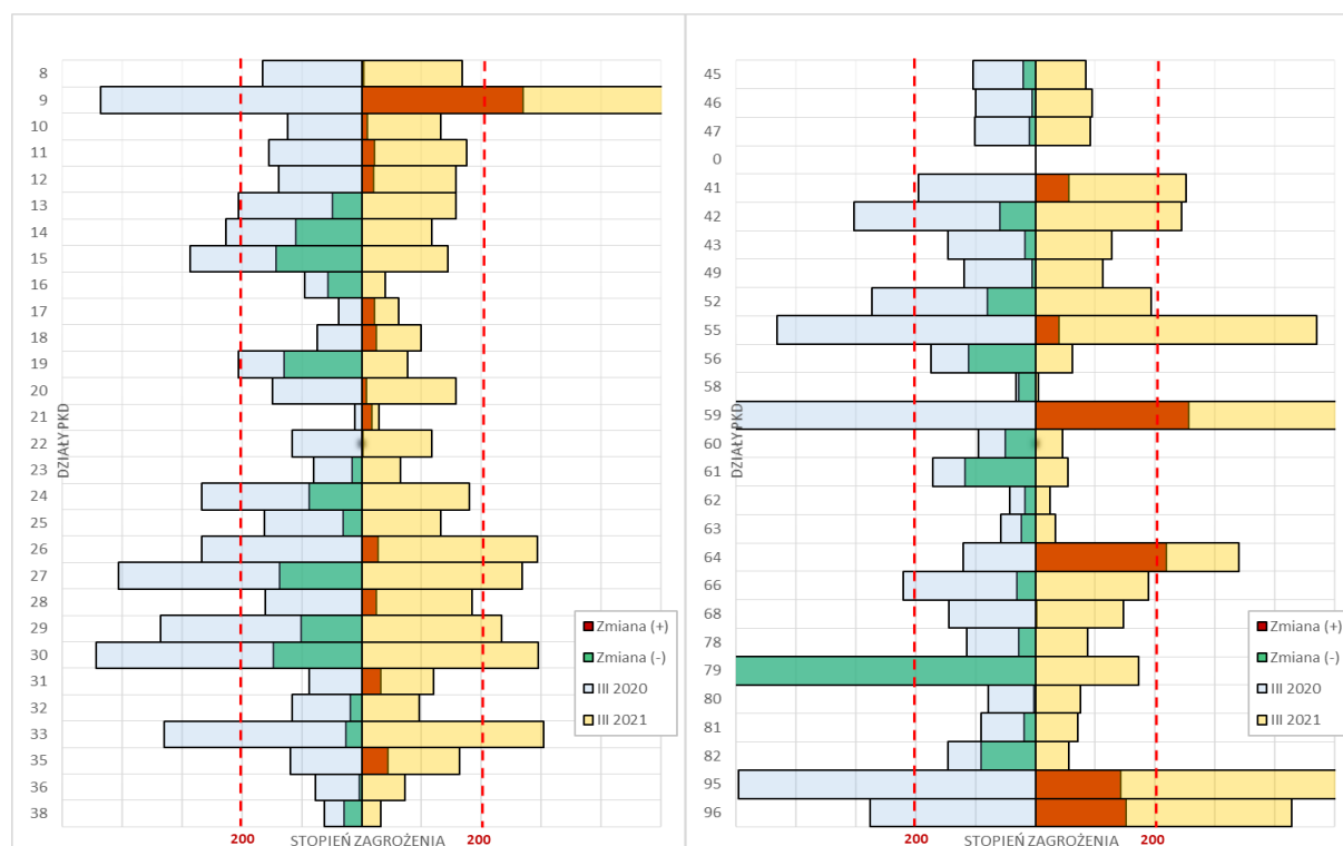
Rysunek 35. Profile zagrożenia upadłością oraz jego zmiany w przedsiębiorstwach dużych według działów PKD w okresie III kw. 2020 r. i III kw. 2021 r.
