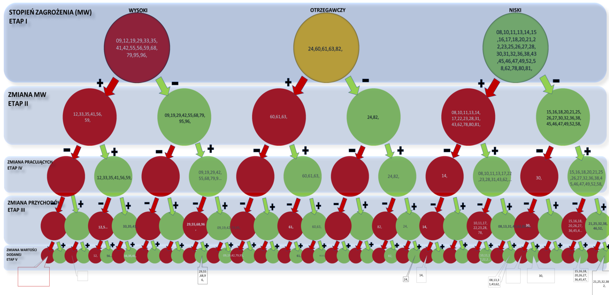
Rysunek 34. Drzewo decyzyjne wyboru działów PKD średnich przedsiębiorstw według stopnia zagrożenia oraz kierunku tempa zmian: stopnia zagrożenia (MW), przychodów ze sprzedaży, pracujących, wartości dodanej według działów PKD w III kw. 2020 r. i w III p. 2021 r.
