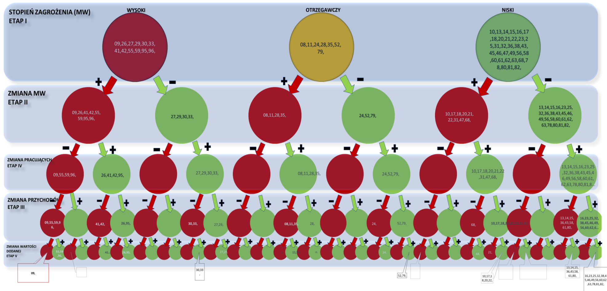
Rysunek 36. Drzewo decyzyjne wyboru działów PKD dużych przedsiębiorstw według stopnia zagrożenia oraz kierunku tempa zmian: stopnia zagrożenia (MW), przychodów ze sprzedaży, pracujących, wartości dodanej według działów PKD w III kw. 2020 r. i III kw. 2021 r.
