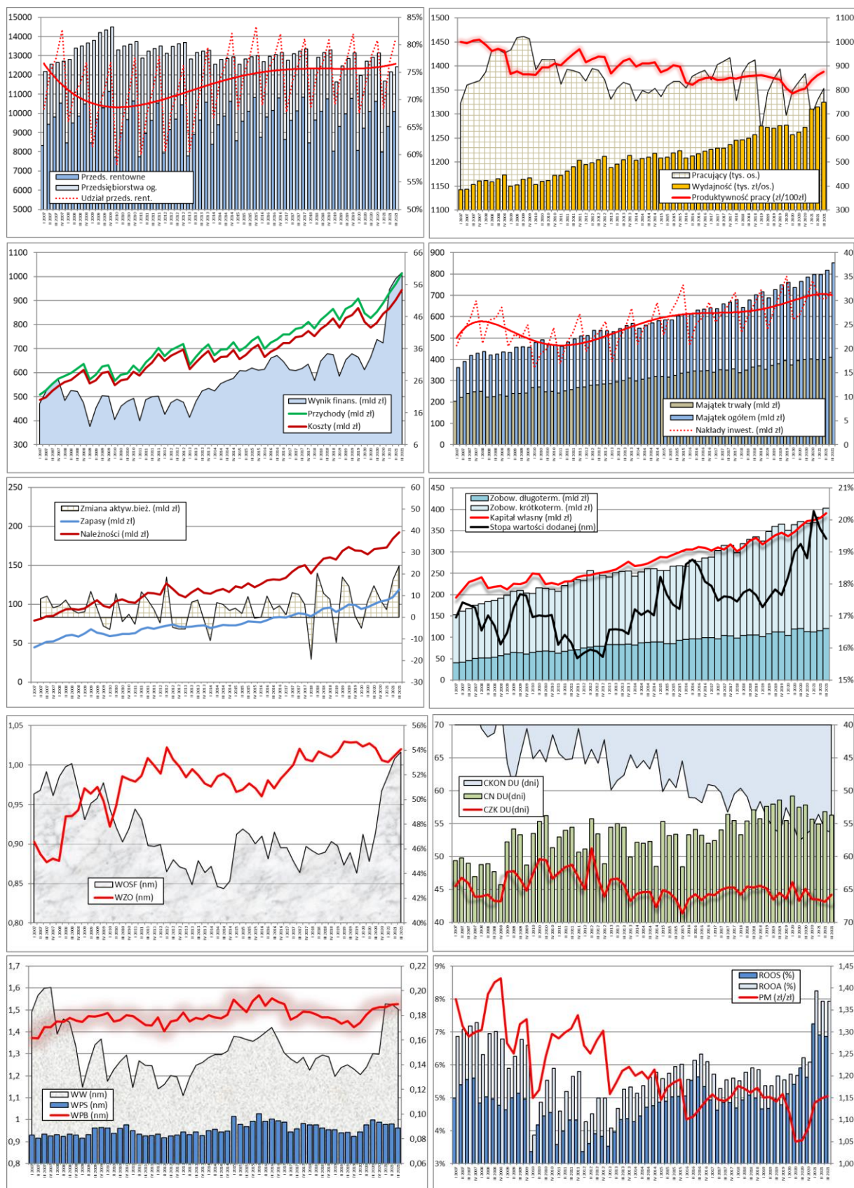
Rysunek 22. Podstawowe charakterystyki przedsiębiorstw średnich (I kw. 2007 r. – III kw. 2021 r.)
