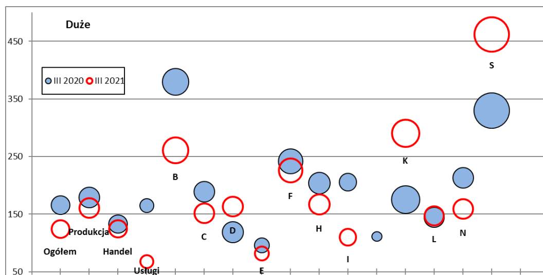
Rysunek 24. Zmiany stopnia zagrożenia upadłością przedsiębiorstw w okresie III kw. 2020 r. – III kw. 2021 r. według rodzaju działalności i sekcji PKD – przedsiębiorstwa duże
