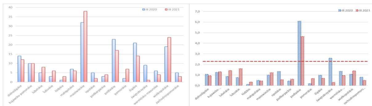
Rysunek 47. Liczba ogłoszonych sądowych postępowań upadłościowych (panel lewy) oraz zmiana Regionalnego Barometru Upadłości (panel prawy) w wybranych województwach w okresie III kw. 2020 r. i III kw. 2021 r.
