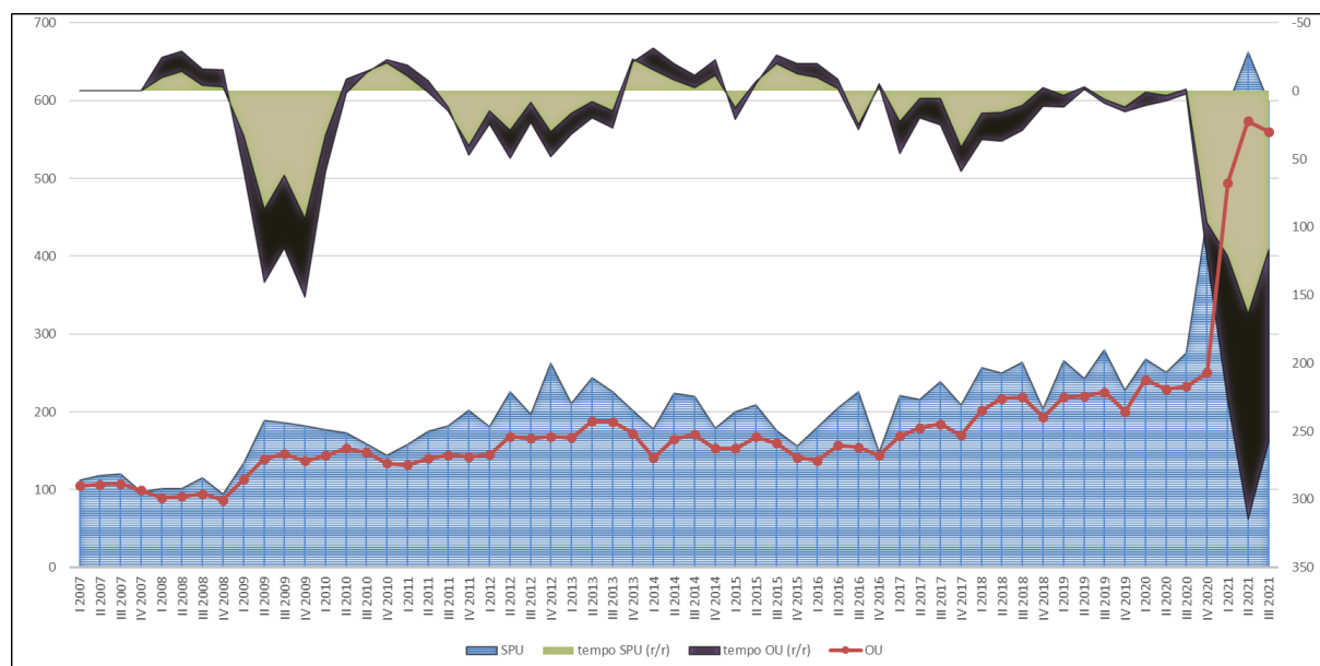
Rysunek 45. SPU i OU oraz tempa ich zmian w okresie I kw. 2007 r. – III kw. 2021 r.
