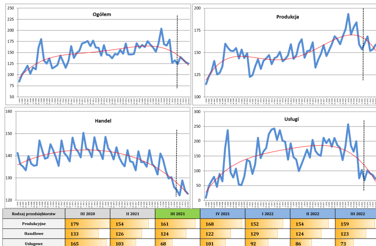
Rysunek 25. Kształtowanie się stopnia zagrożenia upadłością przedsiębiorstw w okresie I kw. 2007 r. – III kw. 2022 r. według rodzaju działalności – przedsiębiorstwa duże
