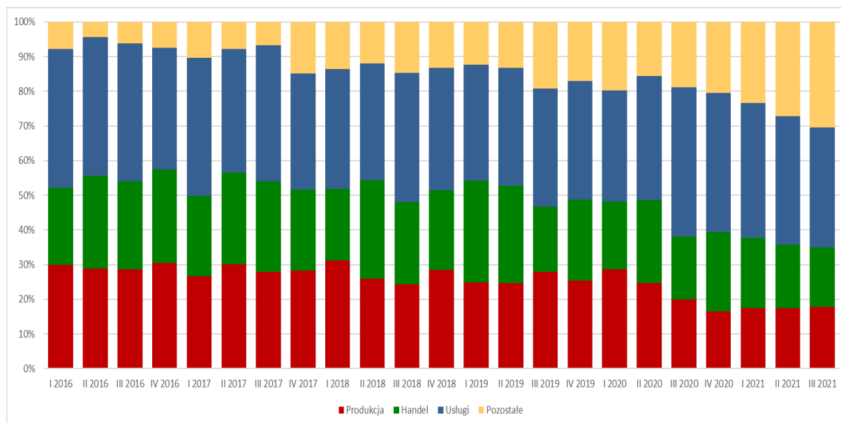
Rysunek 48. Liczba postępowań upadłościowych przedsiębiorstw według rodzaju działalności w okresie I kw. 2016 r. – III kw. 2021 r.
