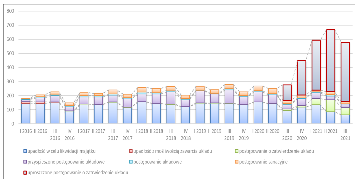
Rysunek 46. Liczba upadłości ze względu na rodzaj postępowania w okresie I kw. 2016 r. – III kw. 2021 r.
