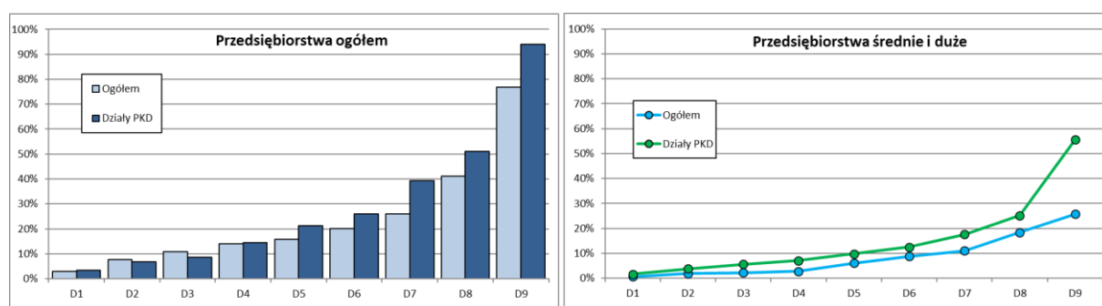
Rysunek 50. Rozkład decylowy wartości bezwzględnej procentowych błędów prognoz stopnia zagrożenia upadłością przedsiębiorstw według zbioru przedsiębiorstw – panel lewy (II p. 2021 r.) oraz średnie i duże – panel prawy (III kw. 2021 r.)
