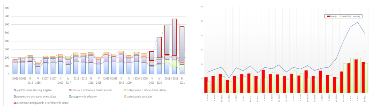
Rysunek 4. Liczba SPU według rodzajów postępowań (panel lewy) oraz według rodzajów prowadzonej działalności (panel prawy) w okresie od I kw. 2016 r. do III kw. 2021 r.
