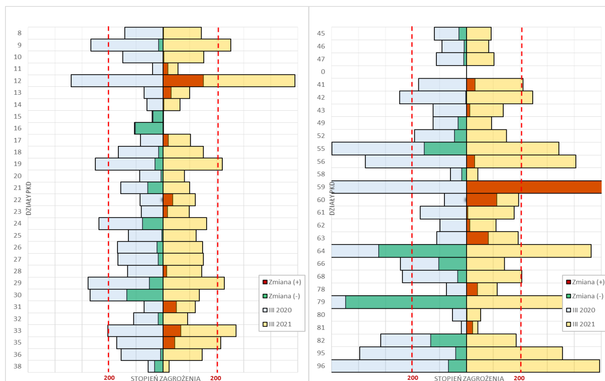
Rysunek 33. Profile zagrożenia upadłością oraz jego zmiany w przedsiębiorstwach średnich według działów PKD w okresie III kw. 2020 r. i III kw. 2021 r.
