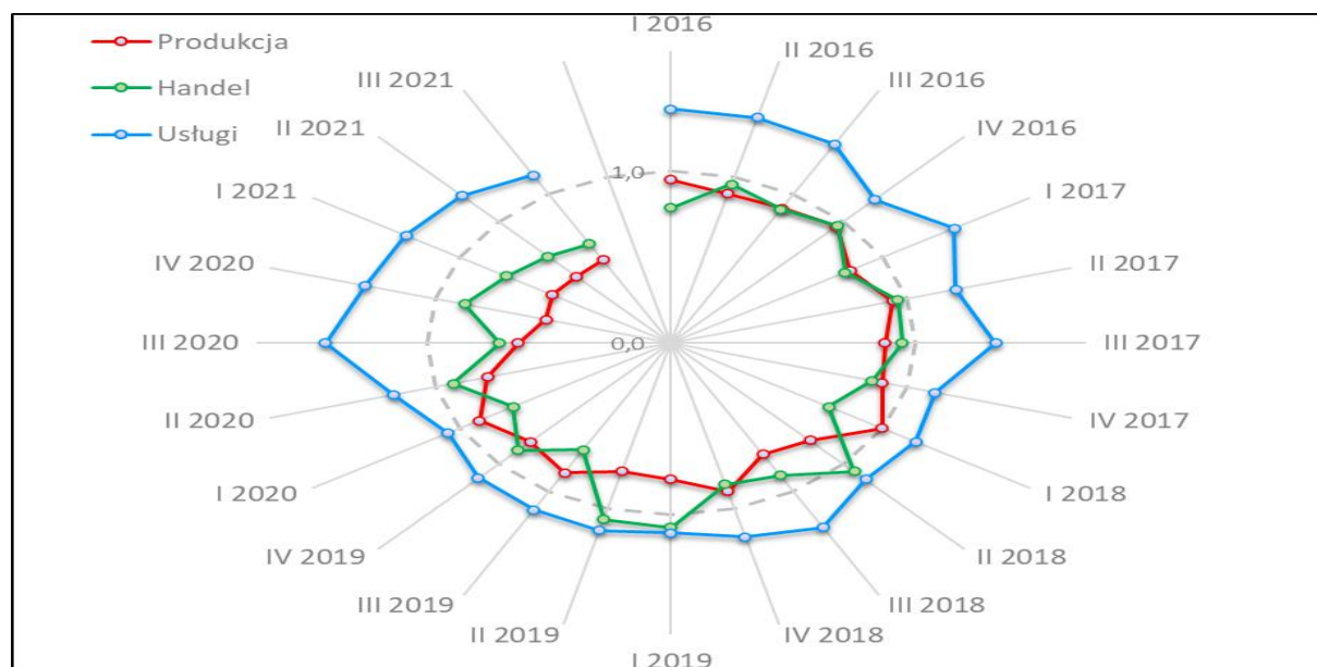
Rysunek 49. Branżowy Barometr Upadłościowy – BBU według rodzaju działalności w okresie I kw. 2016 r. – III kw. 2021 r.
