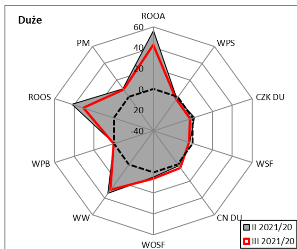
Rysunek 28. Tempo zmian podstawowych wskaźników finansowych przedsiębiorstw w III kw. 2021/ III kw. 2020 r. oraz II kw. 2021/ II kw. 2020 r. (w %, r/r) – przedsiębiorstwa duże
