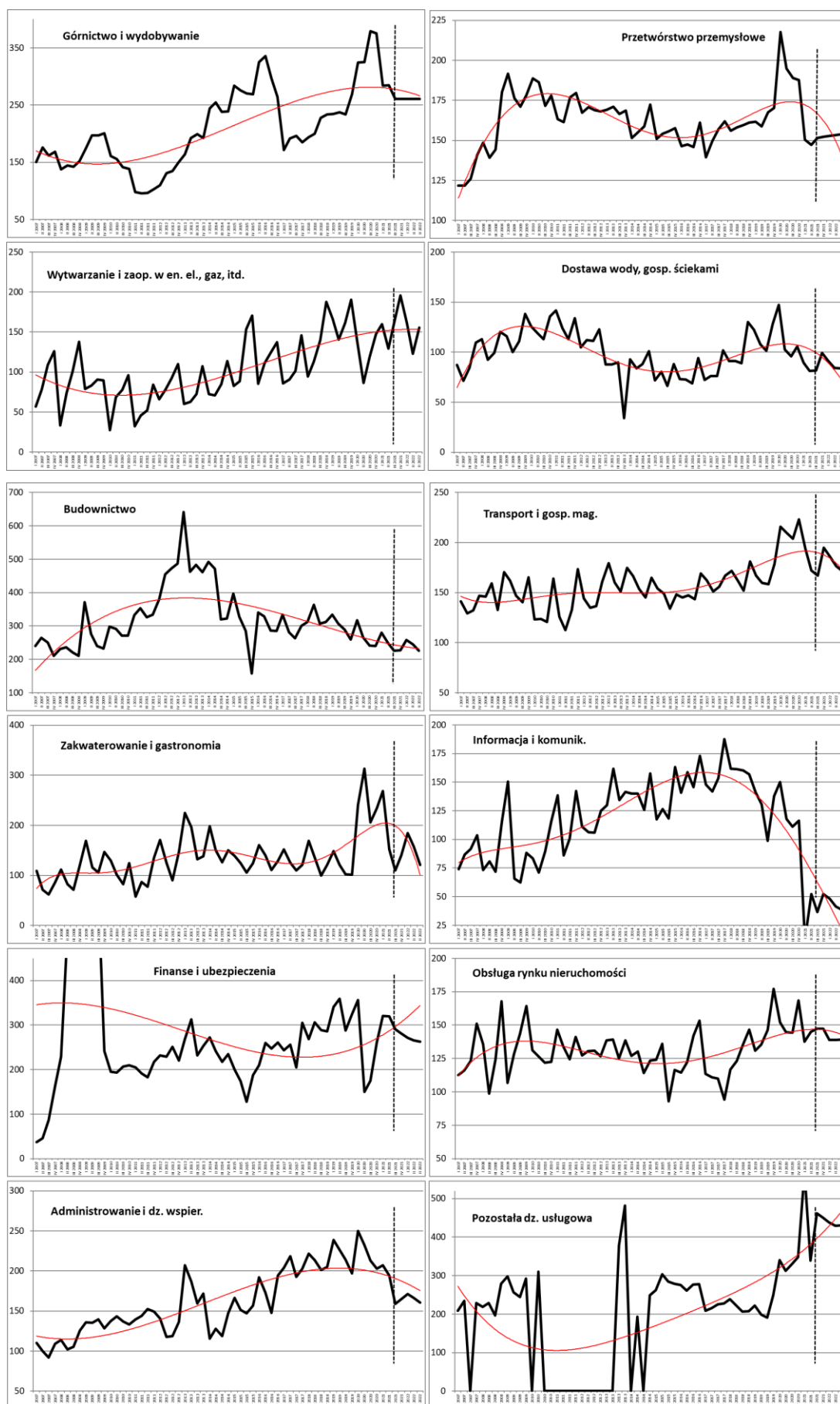
Rysunek 26. Kształtowanie się stopnia zagrożenia upadłością przedsiębiorstw w okresie I kw. 2007 r. – III kw. 2022 r. według sekcji PKD (działów GN) – przedsiębiorstwa duże
