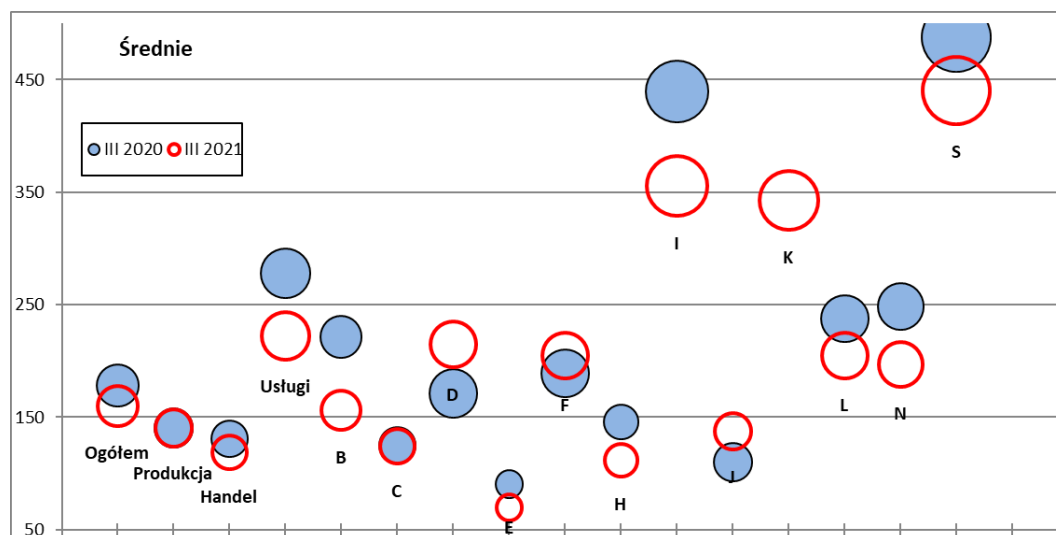
Rysunek 19. Zmiany stopnia zagrożenia upadłością przedsiębiorstw w okresie III kw. 2020 r. – III kw. 2021 r. według rodzaju działalności i sekcji PKD – przedsiębiorstwa średnie
