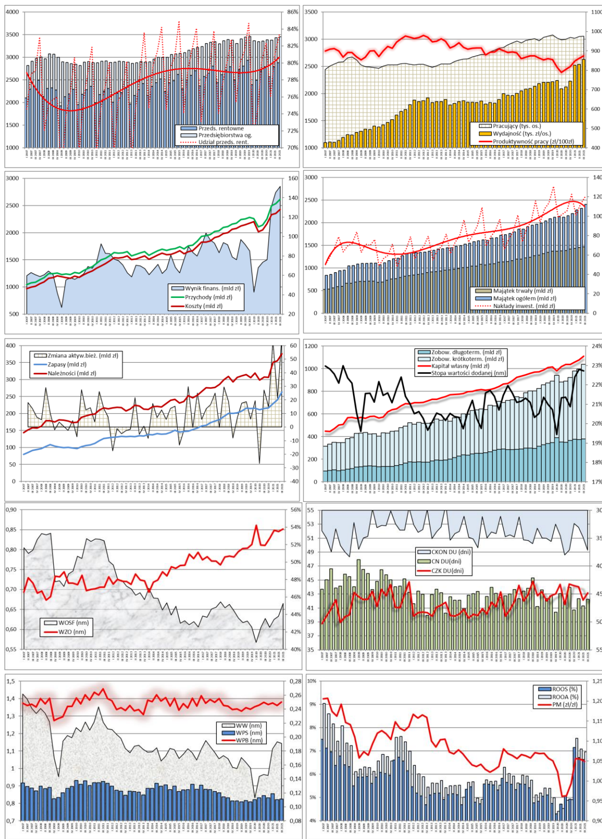
Rysunek 27. Podstawowe charakterystyki przedsiębiorstw dużych (I kw. 2007 r. – III kw. 2021 r.)
