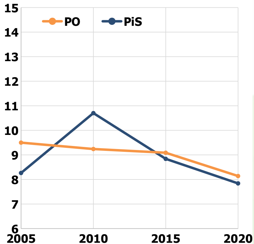
нахили по осі NW-SE
